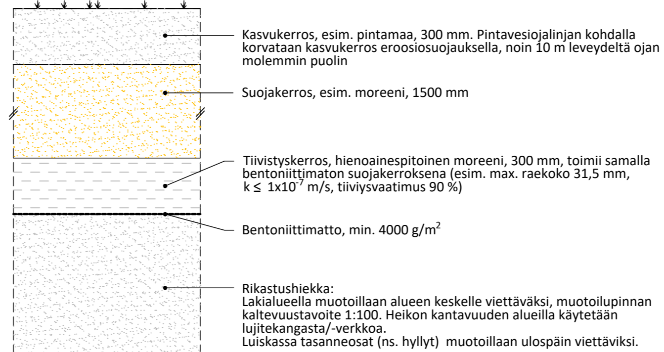
DET6a Pintasulkurakenne, rikastushiekka-allas (1:20)
