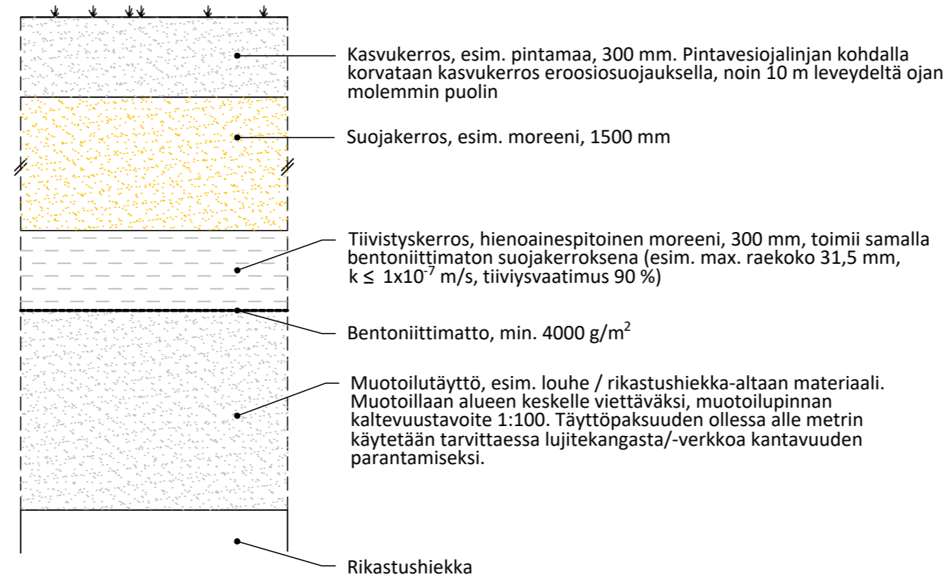
DET6c Pintasulkurakenne, selkeytysallas (1:20)
