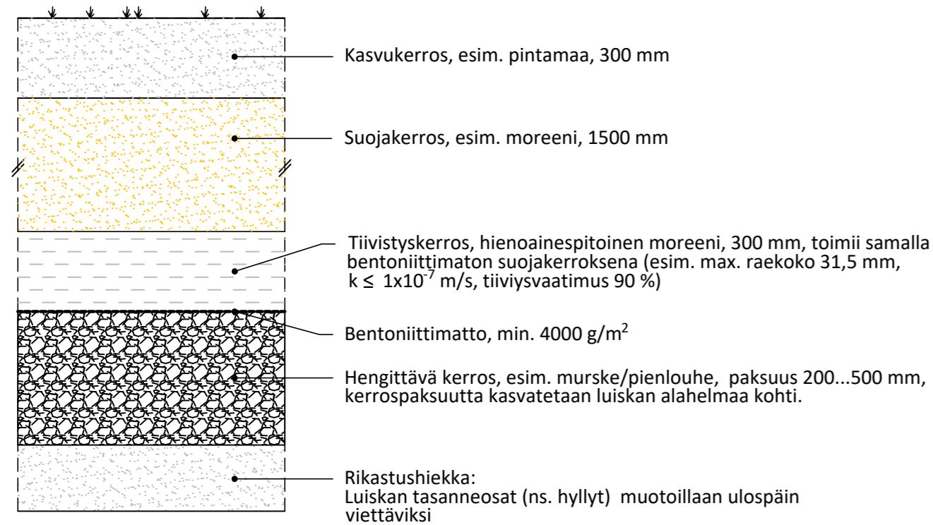
DET6b Pintasulkurakenne, rikastushiekka-allas, luiskan alahelma, ns. hengittävä rakenne (1:20)
