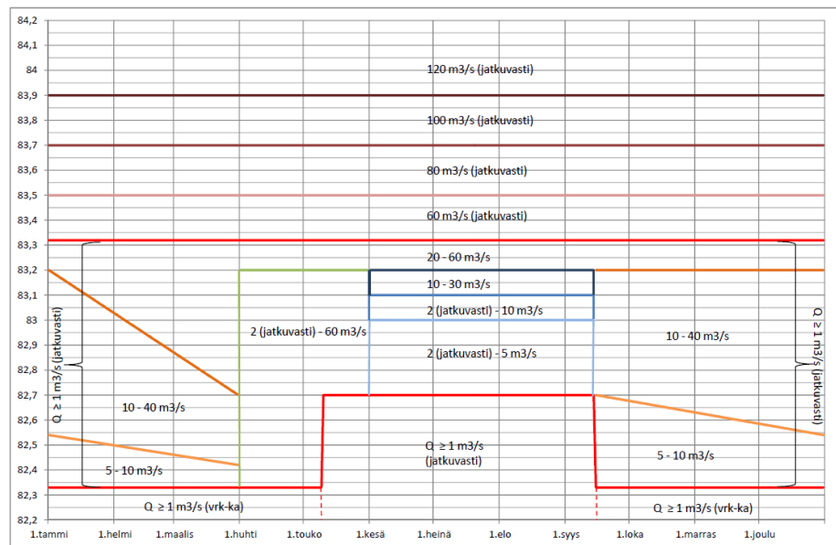
Kuva 1. Kyrösjärven säännöstelykaavio
